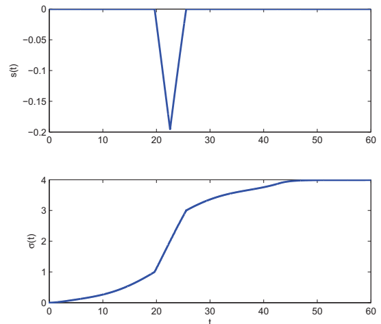
Fig. 6. Steering variable s(t) and parameter \sigma(t) .
